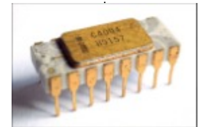
premier microprocesseur 1971
